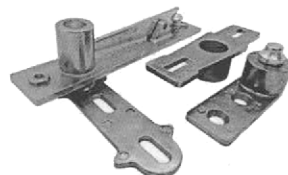
Pivote centrado de Zamac
